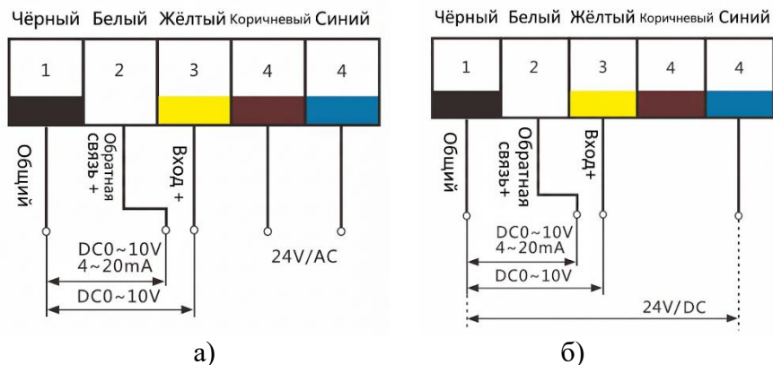
Рисунок 3. Схемы подключения а – 24В переменного тока, б – 24В постоянного тока
