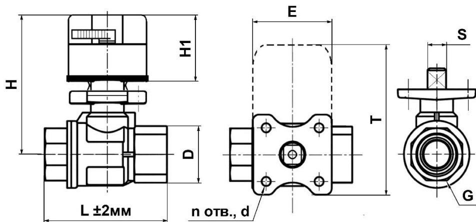
Рисунок 2 – Размеры изделия
