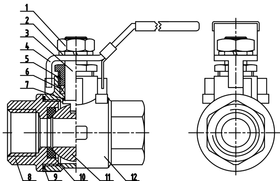
Рисунок 2 - Составные части изделия
