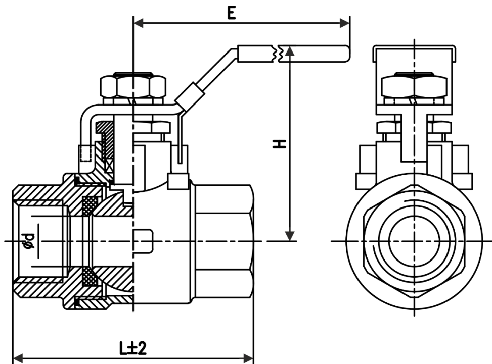
Рисунок 3 - Размеры изделия
