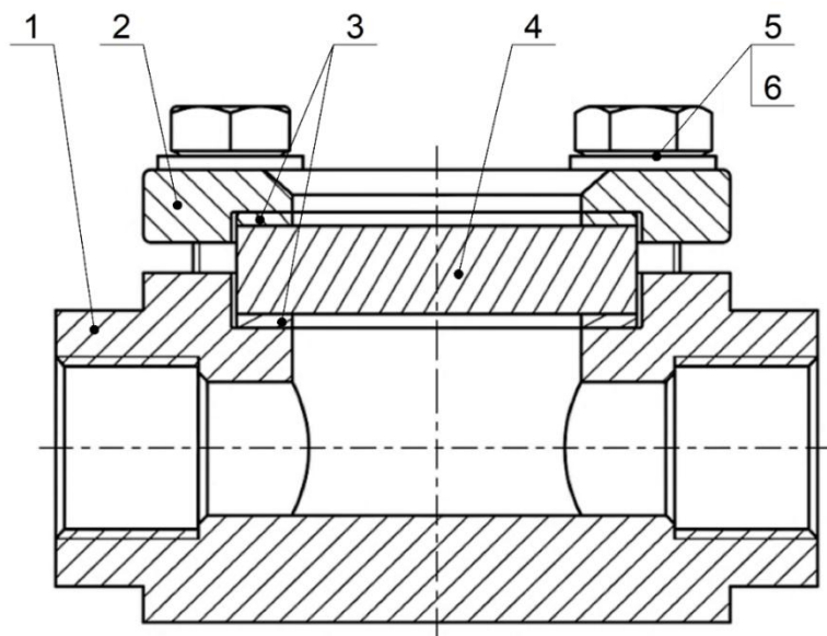
Рисунок 2 – Составные части изделия
