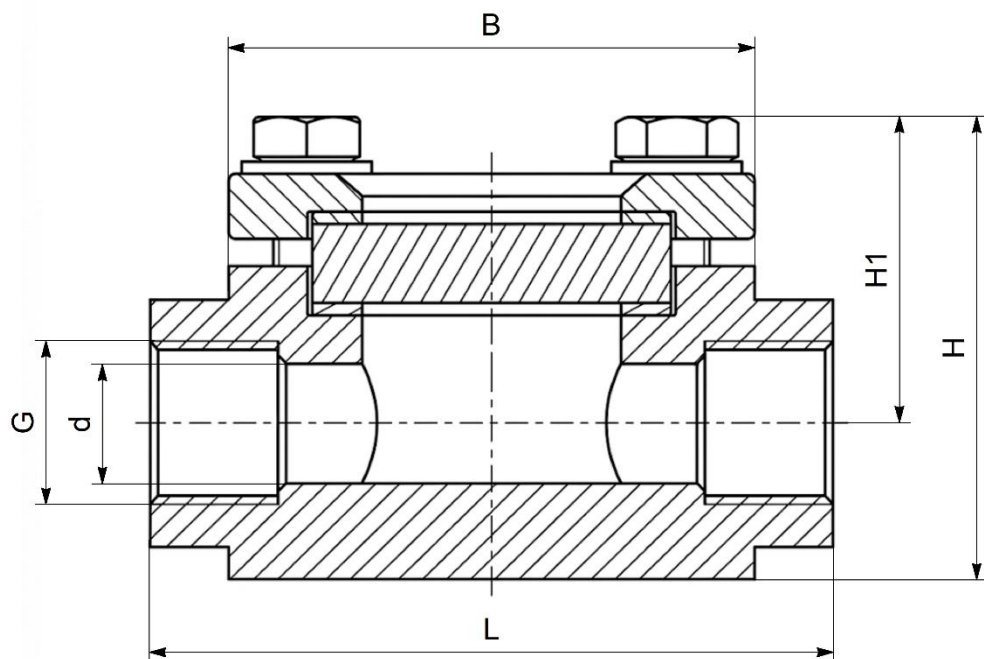
Рисунок 3 – Размеры изделия
