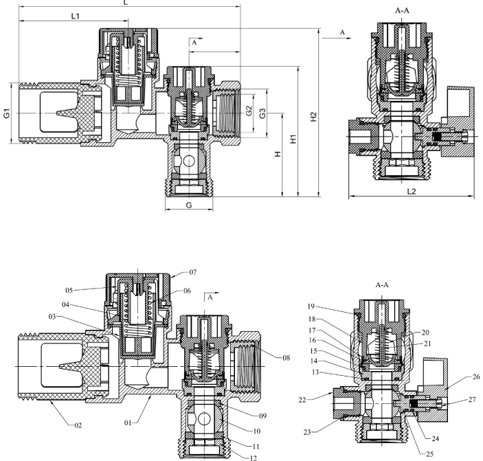
Рис. 1 Группа безопасности для водонагревателя.
