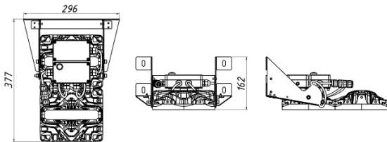
Рисунок 1 Общий вид светильника «L-pixel 2 Em banner» Поворотное крепление
