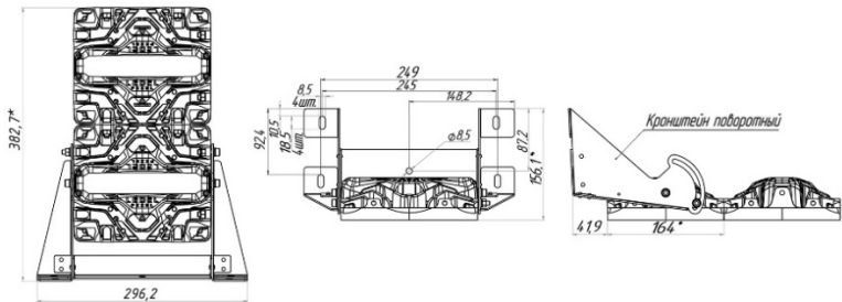
Рисунок 1 Общий вид светильника «L-pixel 2 banner» Поворотное крепление
