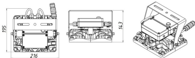
Рисунок 1 Общий вид светильника «L-pixel 1 Em banner» Поворотное крепление
