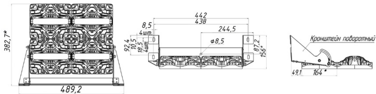
Рисунок 1 Общий вид светильника «L-pixel 4 banner» Поворотное крепление
