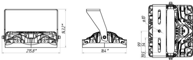
Рисунок 1 Общий вид светильника «L-pixel 1 banner» Поворотное крепление
