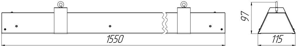
Рисунок 1. Светильник FLL
