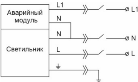
Рисунок 2. Схема подключения светильника
