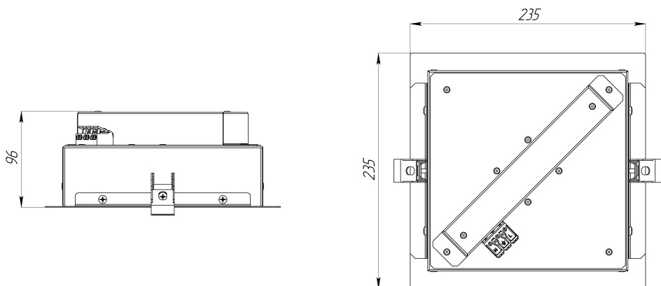
Рисунок 1. Светильник ДВО 02
