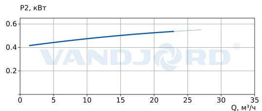
VSL - Канализационные насосы с закрытым рабочим колесом
