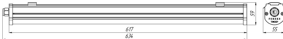
Рисунок 1. Светильник ДСО 2.0
