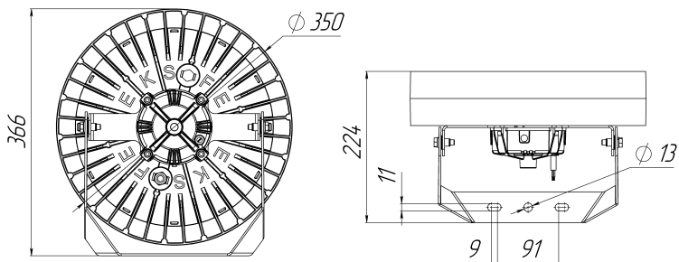
Рисунок 2. Светильник Wheel с кронштейном
