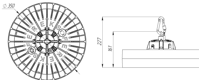
Рисунок 1. Светильник Wheel с подвесным креплением
