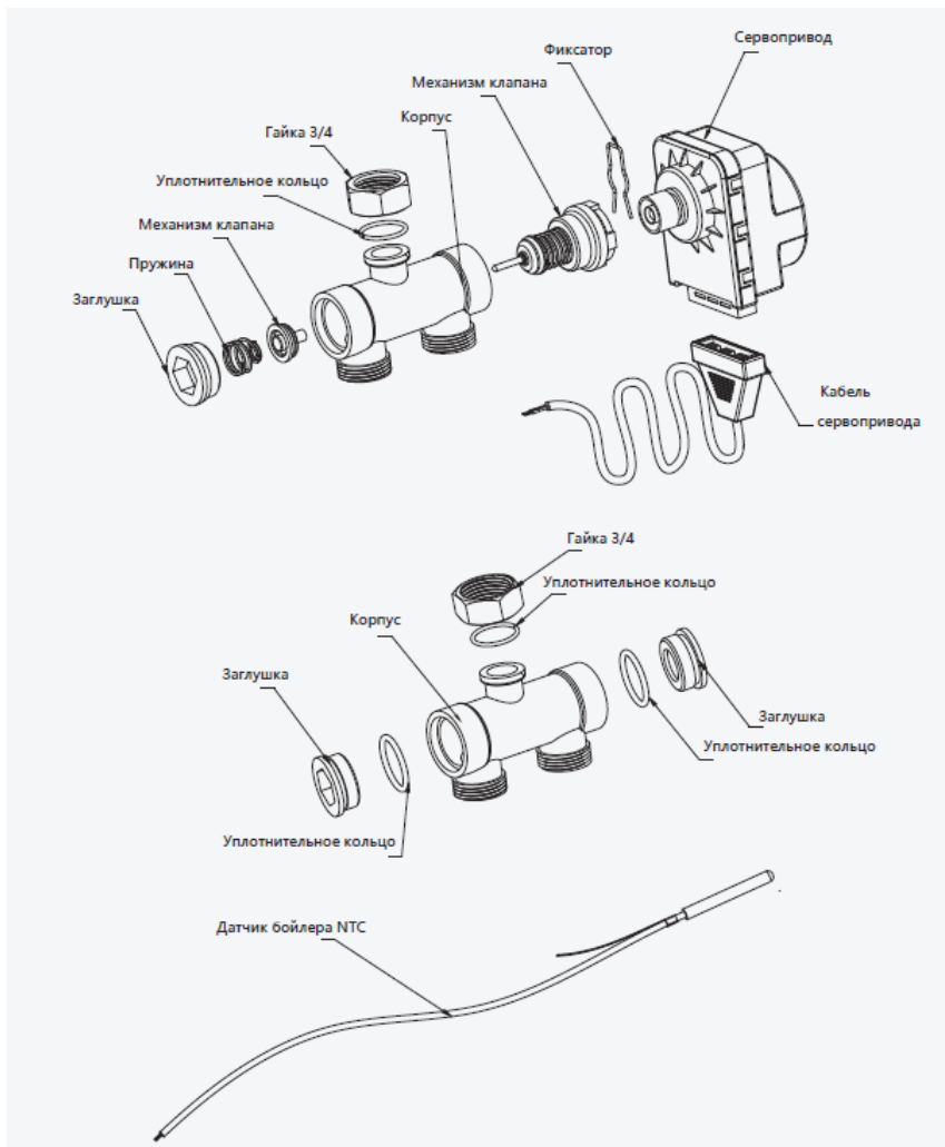
Рисунок 3. Конструкция комплекта трехходового клапана
