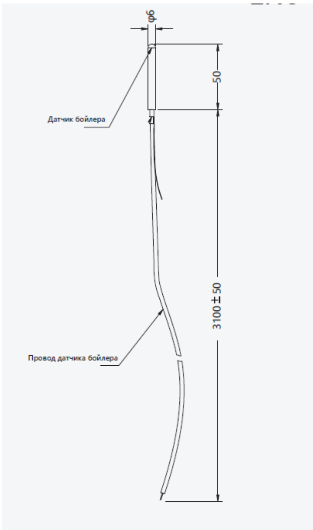
Рисунок 4. Конструкция погружного датчика бойлера NTC
