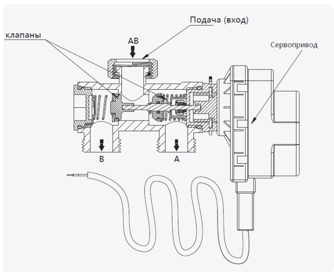
Рисунок 1. Принцип работы
