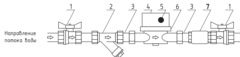
Рис. 1 Рекомендуемая схема установки счётчика:
