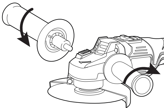
Рисунок 2.2.5. Установка боковой рукоятки
