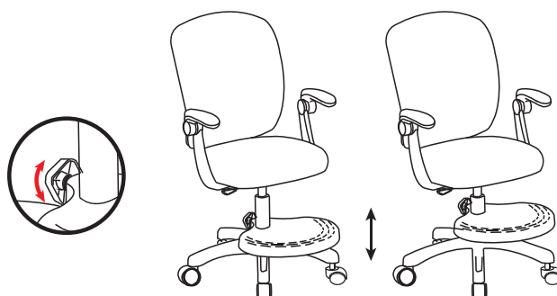
Регулировка высоты подставки для ног / Height of the footrest adjustment / Аяқ тіреуішінің биіктігін реттеу
