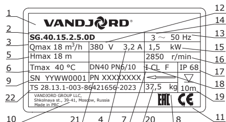
Рис. 2 Фирменная табличка
