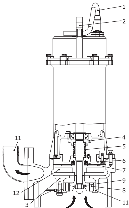
Рис. 1 Насос SG
