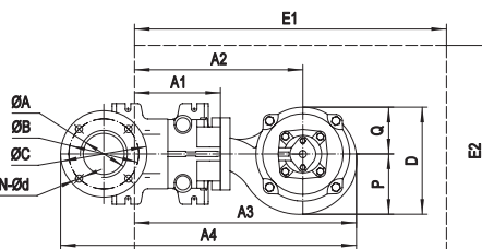
Фланец напорного патруб­ка насоса SG.50 PN6/ PN10
