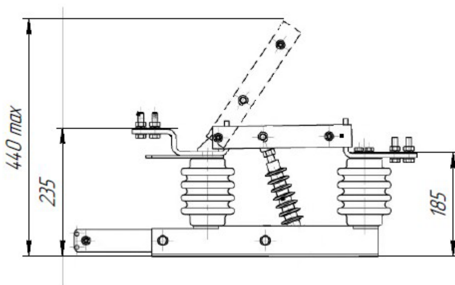
Габаритные и установочные размеры РВЗ.16-10/1000 УХЛ2
