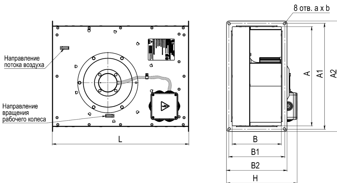
Рисунок 1. Габаритные и присоединительные размеры ВКП
