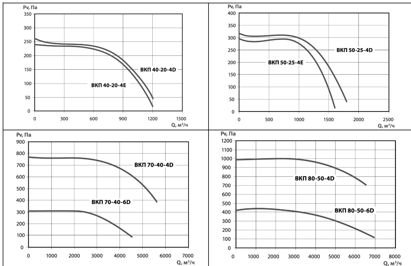
Рисунок 3. Аэродинамические характеристики вентиляторов канальных прямоугольных с вперед загнутыми лопатками (статическое давление от производительности)
