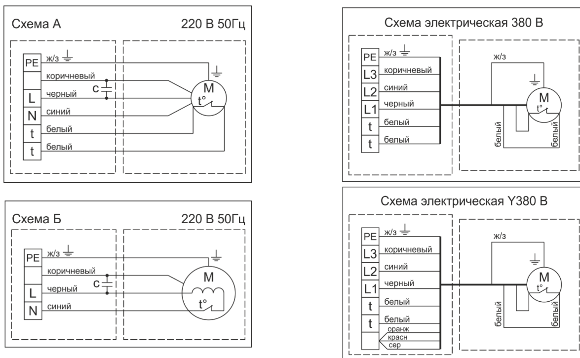
Рисунок 2. Схемы подключения вентилятора ВКП
