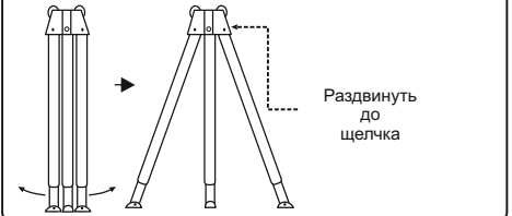
Рис. 3. Фиксация опор
