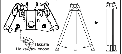
Рис. 5. Регулировка высоты
