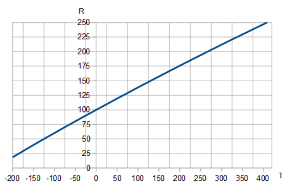
Рисунок А.2 – График зависимости сопротивления от температуры
