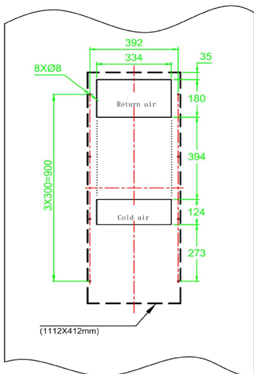
Рис. 1 - Размер для вырезания двери
