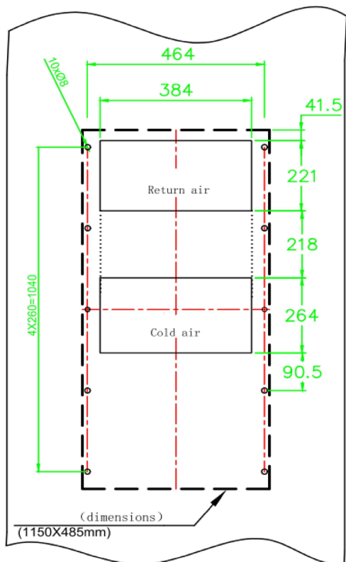
Рис. 1 - Размер для вырезания двери
