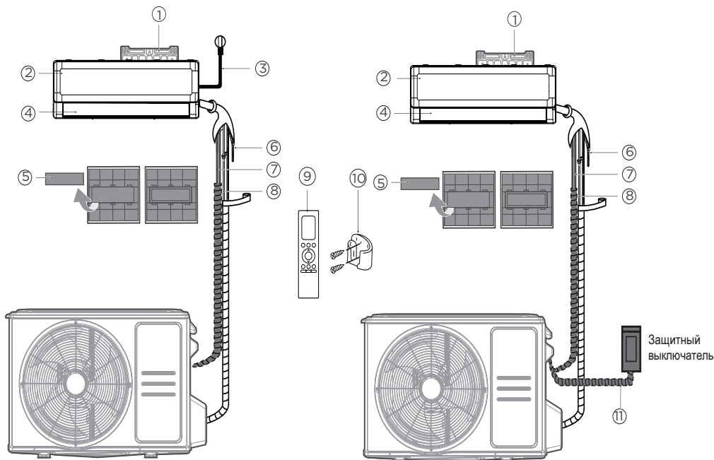
Модели с электропитанием от внутреннего блока
