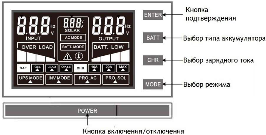
Рис.3 Панель управления
