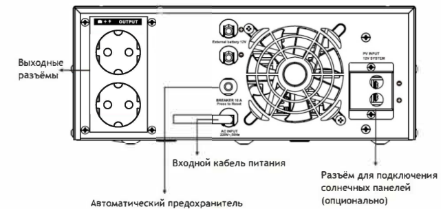
Рис.1 Задняя панель
