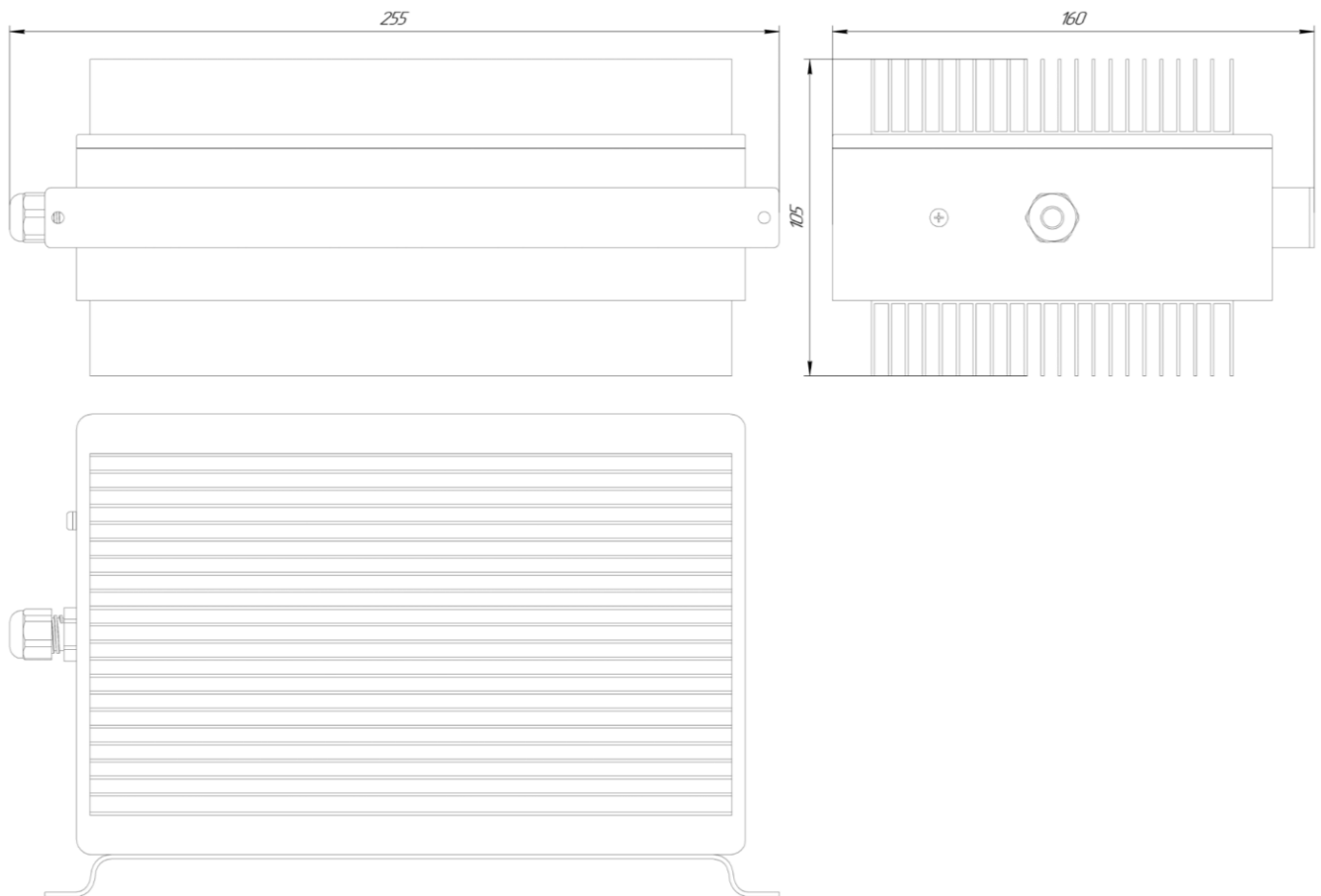
Рисунок А.2 – Габаритные размеры
