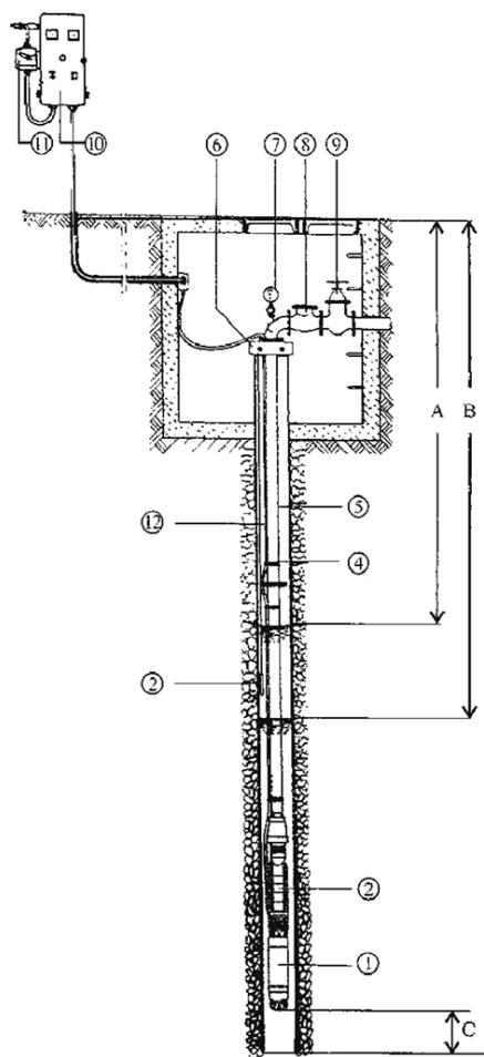
Схема подключения насоса
