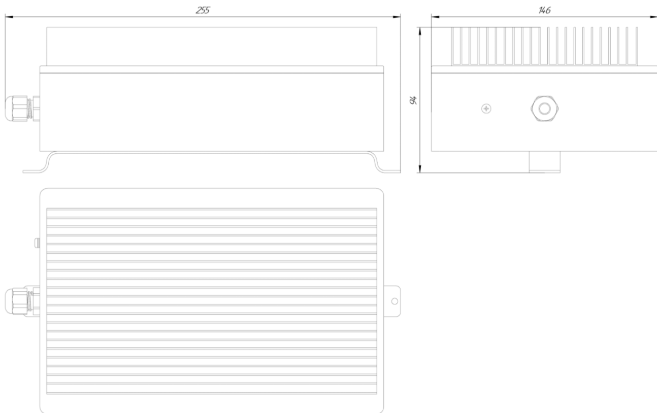
Рисунок А.2 – Габаритные размеры
