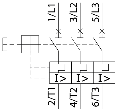
Выключатели OptiStart ME GV2ME, OptiStart ME GV3ME
