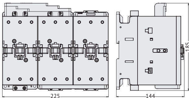
FX-3431
