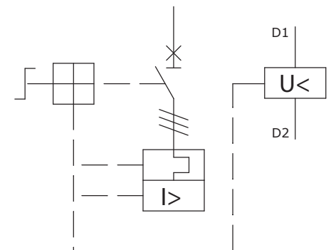
Расцепитель минимального напряжения MP-U...-T2
