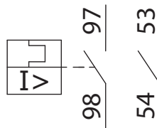
Контакт вспомогательный поперечный OptiStart ME CVAE20
