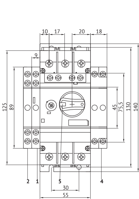
Автоматические выключатели MP-63R...-T2
