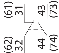
Контакт вспомогательный боковой OptiStart ME CVAN11
