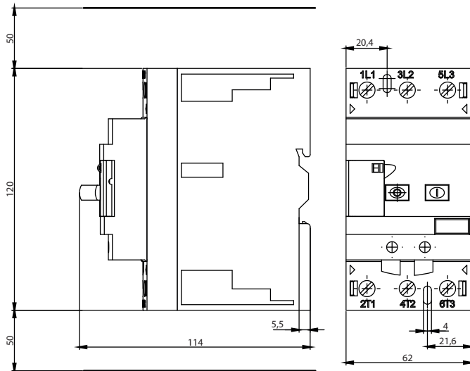
GV3ME
