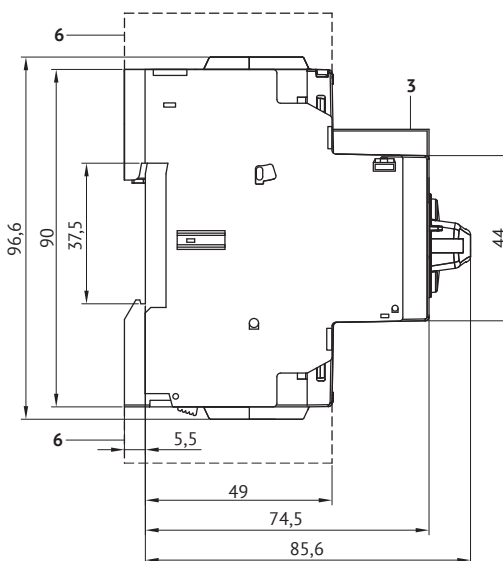
Автоматические выключатели MP-32RH...-T2 и MP-32RH1...-T2
