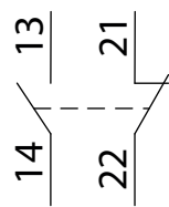
Контакт вспомогательный боковой OptiStart ME CV3A01
