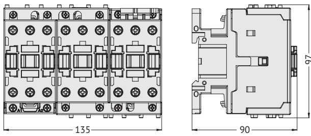
FX-3231
