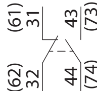
Контакт мгновенного действия CVAN11
