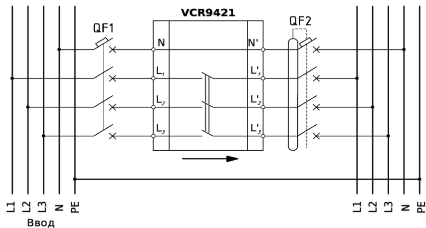
Рисунок 1 – Принципиальная схема подключения реле контроля напряжения и тока VCR9421
