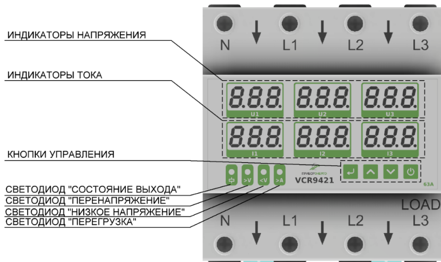
Рисунок 2 – Лицевая панель реле контроля напряжения и тока VCR9421
