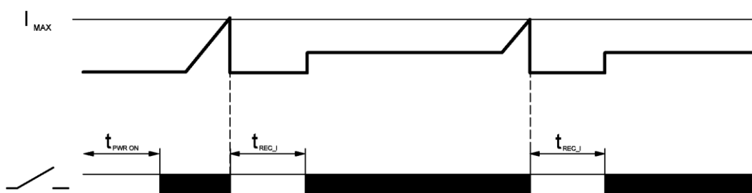
Рисунок 4 – Диаграмма работы реле контроля напряжения и тока VCR9421, срабатывание по току
