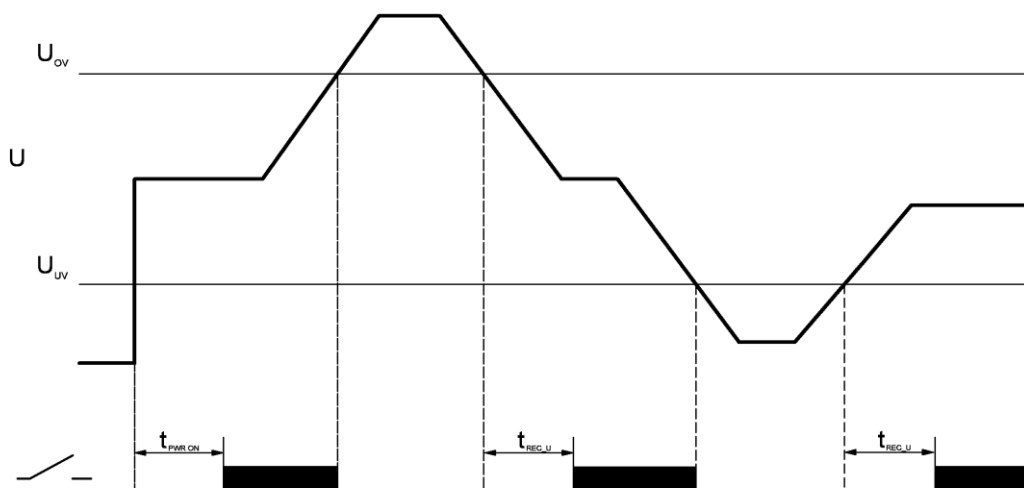
Рисунок 3 – Диаграмма работы реле контроля напряжения и тока VCR9421, срабатывание по напряжению
