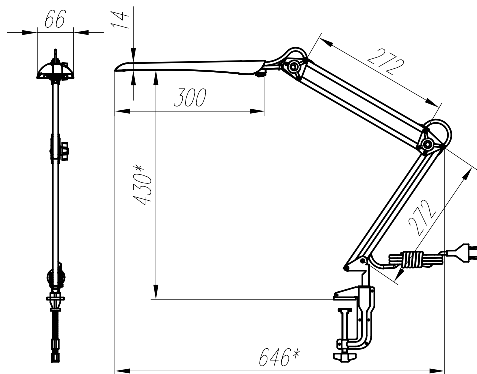
Внешний вид светильника ПДБ57-8-004 "Гермес"
