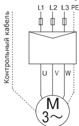
Прямой пуск (3-проводная схема)
