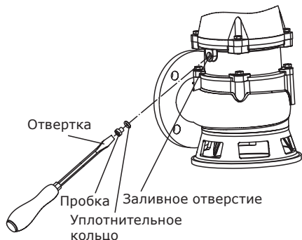
Рис. 13 Отверстие для слива и заливки масла
