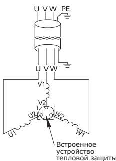
Прямой пуск (3-проводная схема)
