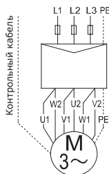
Прямой пуск (6-проводная схема)
