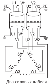
Прямой пуск (6-проводная схема)
