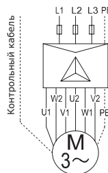
Пуск «Звезда-треугольник» (6-проводная схема)
