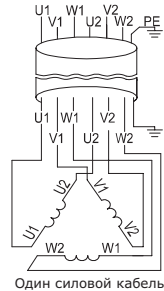
Пуск «Звезда-треугольник» (6-проводная схема)
