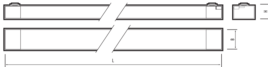
Рис.1 Прожектор PTR 19
