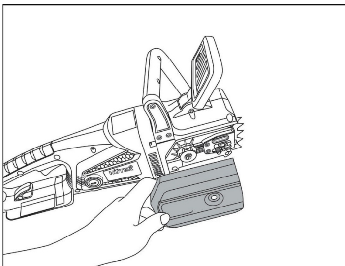
Рис. 2. Снятие прижимной крышки шины
