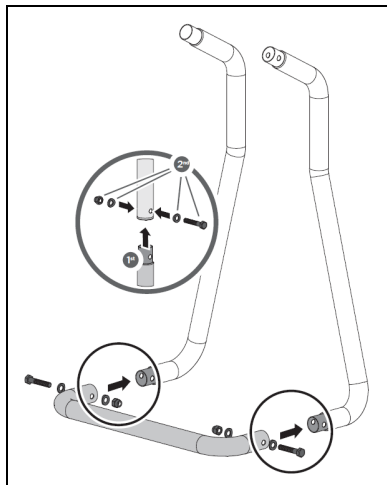
Рис. 3. Сборка передней опоры
