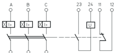
Рисунок 5.19 – Трехполюсный выключатель с электромагнитными расцепителями, независимым расцепителем и с одним размыкающим вспомогательным контактом
