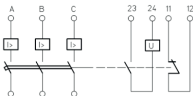
Рисунок 5.20 – Однополюсный выключатель в трехполюсном корпусе с электромагнитными расцепителями с гидравлическим замедлением, с одним замыкающим и одним размыкающим вспомогательными контактами
