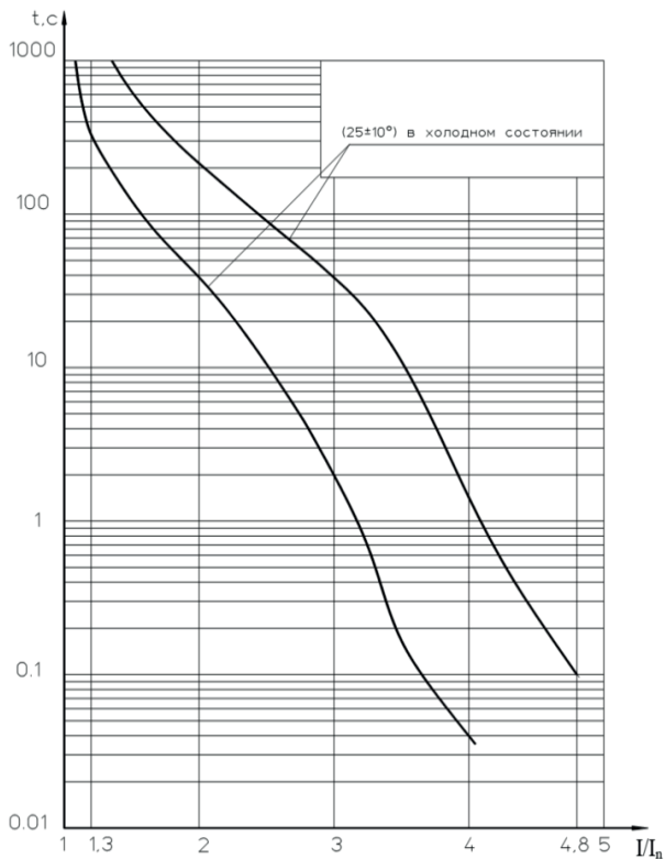
Рисунок Г.1 – Выключатель с уставкой по току срабатывания 4I_n
