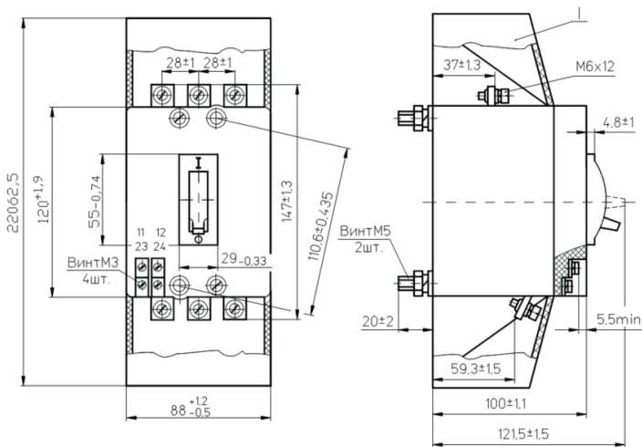
Рисунок Б.6 – Сверление отверстий под винты крепления трехполюсного выключателя:
