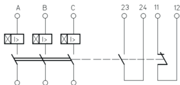
Рисунок Б.15 – Трехполюсный выключатель с электромагнитными расцепителями, с одним замыкающим и одним размыкающим вспомогательными контактами
