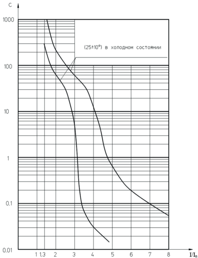
Рисунок Г.2 – Выключатель с уставкой по току срабатывания 6 I_n
