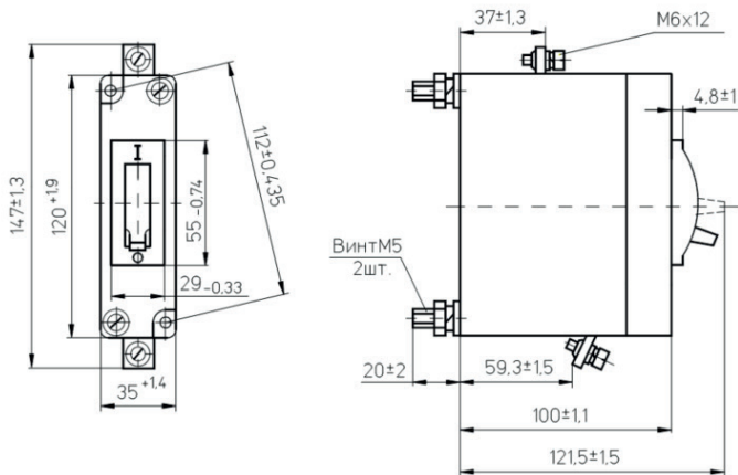
Рисунок Б.1 – Однополюсный выключатель
