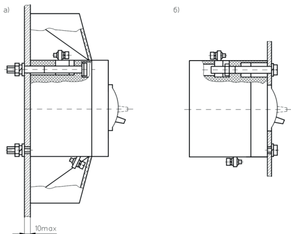
Рисунок Б.10 – Крепление выключателя в пластмассовой оболочке: а) на панели; б) за панелью.
