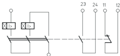
Рисунок 5.21 – Однополюсный выключатель в трехполюсном корпусе с электромагнитными расцепителями, с одним замыкающим и одним размыкающим вспомогательными контактами
