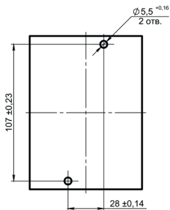
Рисунок Б.6 – Сверление отверстий под винты крепления трехполюсного выключателя:
