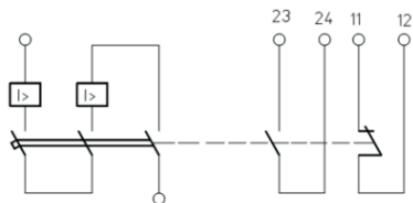
Рисунок 5.21 – Однополюсный выключатель в трехполюсном корпусе с электромагнитными расцепителями, с одним замыкающим и одним размыкающим вспомогательными контактами
