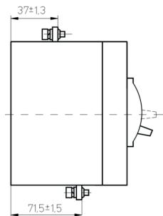
Рисунок Б.10 – Крепление выключателя в пластмассовой оболочке: а) на панели; б) за панелью.
