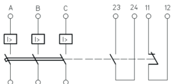
Рисунок Б.16 – Трехполюсный выключатель с электромагнитными расцепителями с гидравлическим замедлением срабатывания, с двумя замыкающими и двумя размыкающими вспомогательными контактами
