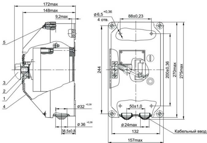
Рисунок Б.12 – Двухполюсный и трехполюсный выключатель в дополнительной оболочке Масса не более 3,5 кг
