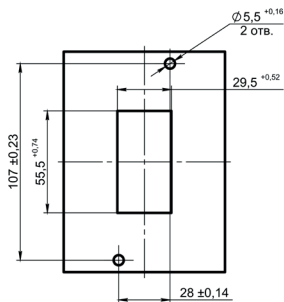
Рисунок Б.6 – Сверление отверстий под винты крепления трехполюсного выключателя:
