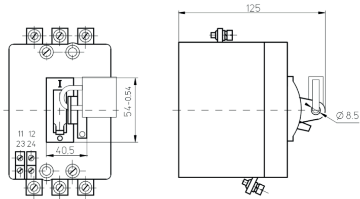
Рисунок Б.12 – Двухполюсный и трехполюсный выключатель в дополнительной оболочке Масса не более 3,5 кг
