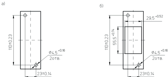
Рисунок Б.2 – Сверление отверстий под винты крепления однополюсного выключателя:
