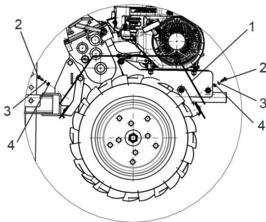
Рис. 5. Установка защитных крыльев.
