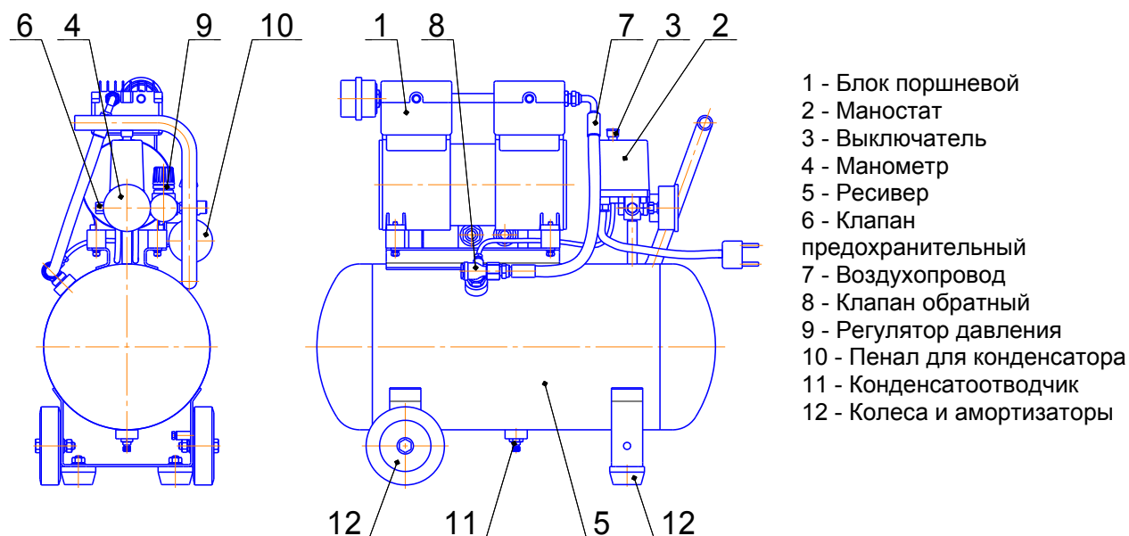
Рисунок 4 - Общий вид компрессора PG-600
