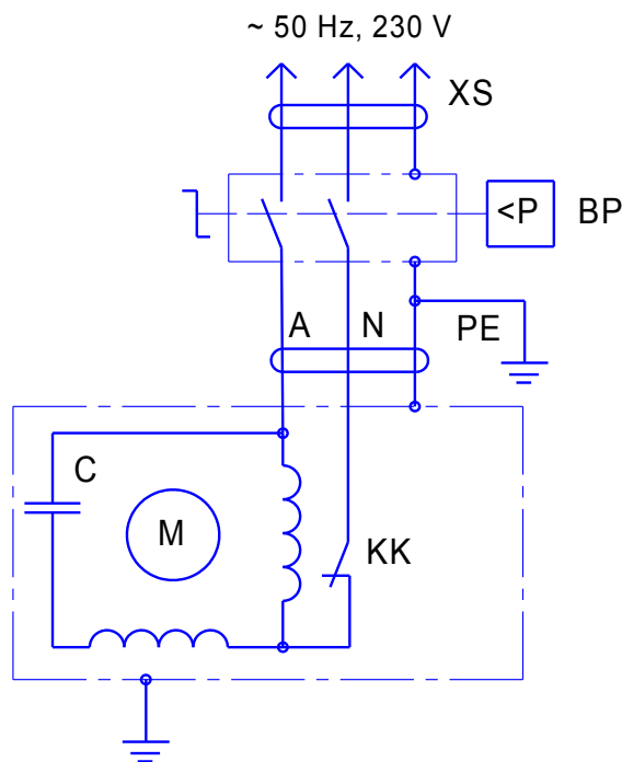
Рисунок А.1 - Схема электрическая принципа
