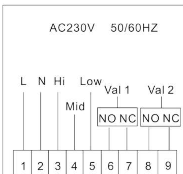
TGT70-AC4, TGT70WIFI-AC4
