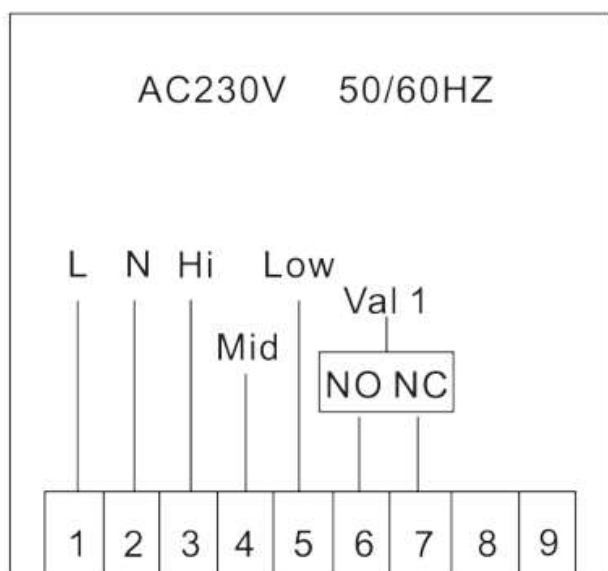
TGT70-AC2, TGT70WIFI-AC2
