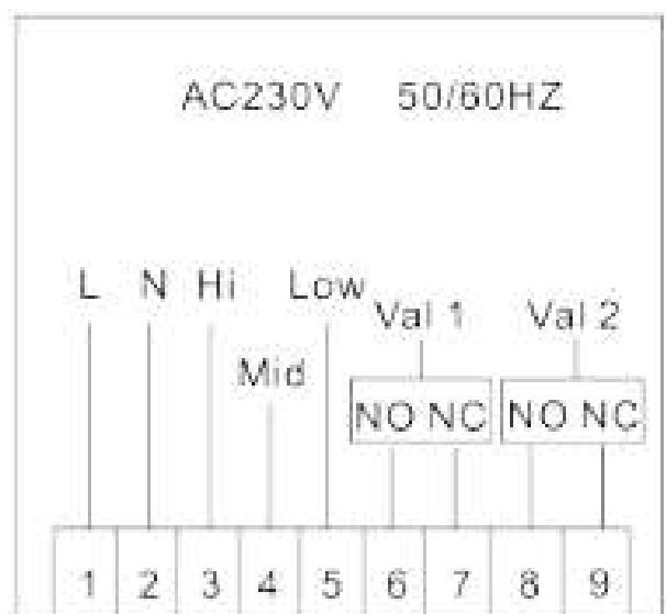
TGT70-AC4, TGT70WIFI-AC4
