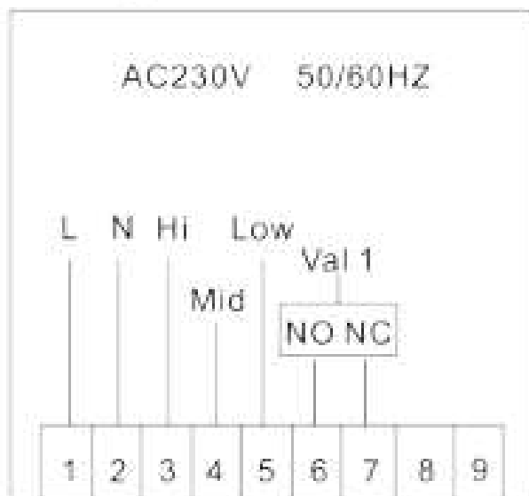
TGT70-AC2, TGT70WIFI-AC2
