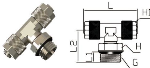
Тройник с накидной гайкой серии КМВВТ-G
