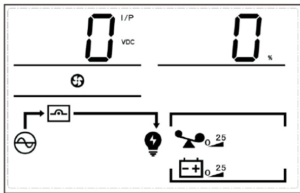
Экран 3: Напряжение АКБ и уровень заряда
