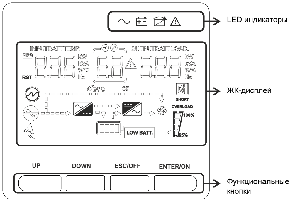
Рисунок 8 – Общий вид органов управления и индикации
