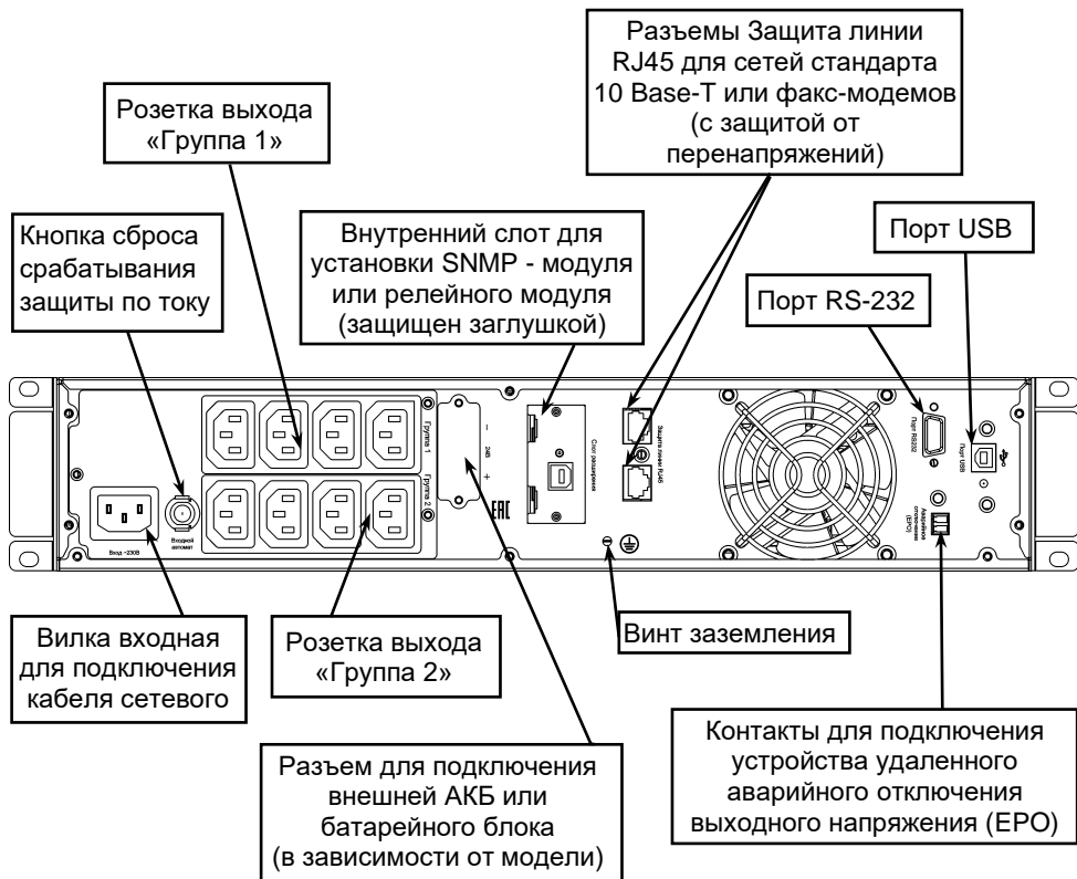
Рисунок 3 – Общий вид задней панели SKAT-UPS 1000-RACK-ON-2x9-E P3, SKAT-UPS 1000-RACK-ON-E P3, SKAT-UPS 1500-RACK-ON-3x9-E P3, SKAT-UPS 1500-RACK-ON-E P3
