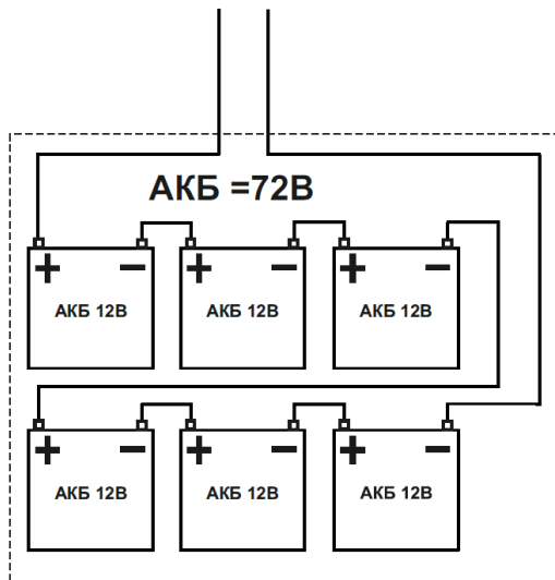
Схема монтажа аккумуляторной батареи для SKAT-UPS 1500-RACK-ON P3 и SKAT-UPS 1500-RACK-ON-E P3
