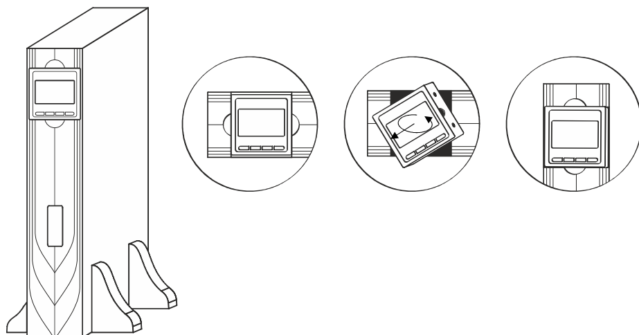
Рисунок 11 – Поворот ЖК-дисплея при напольной установке
