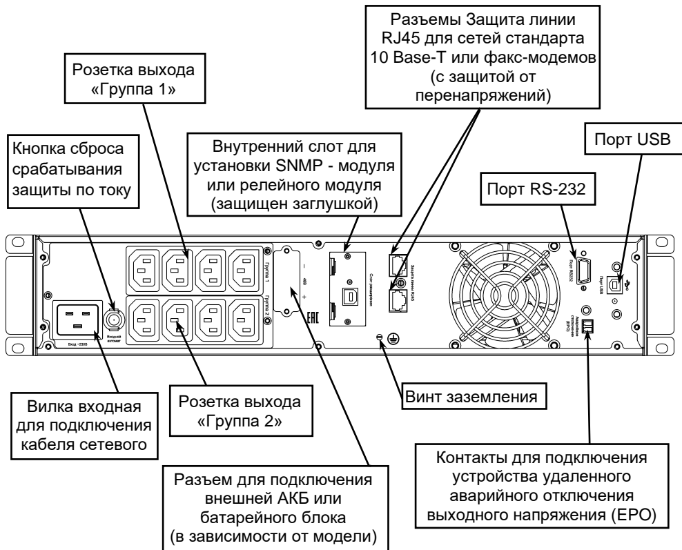
Рисунок 5 – Общий вид задней панели SKAT-UPS 2000-RACK-ON-4x9 P3, SKAT-UPS 2000-RACK-ON P3
