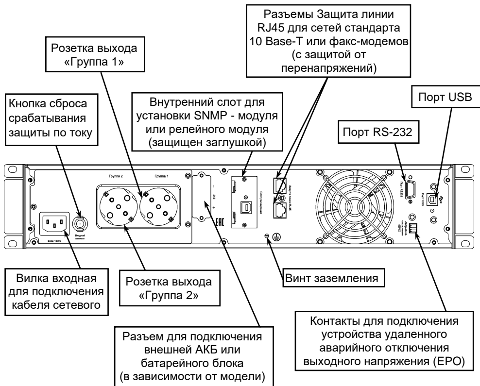
Рисунок 2 – Общий вид задней панели SKAT-UPS 1000-RACK-ON-2x9 P3, SKAT-UPS 1000-RACK-ON P3, SKAT-UPS 1500-RACK-ON-3x9 P3, SKAT-UPS 1500-RACK-ON P3
