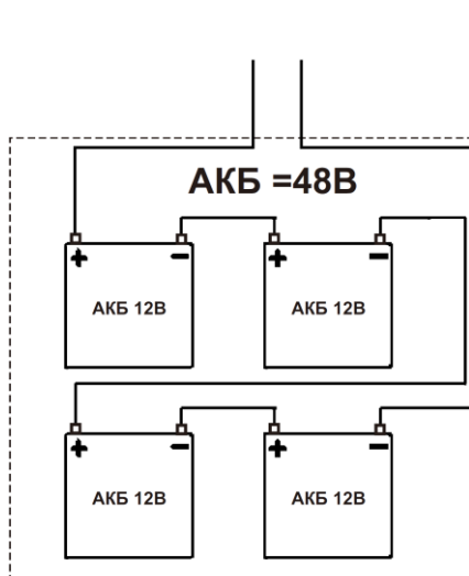
Схема монтажа аккумуляторной батареи для SKAT-UPS 1000-RACK-ON P3 и SKAT-UPS 1000-RACK-ON-E P3
