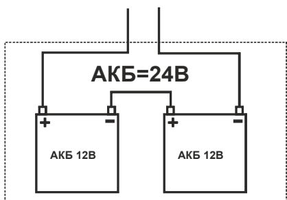
Схема монтажа аккумуляторной батареи для SKAT-UPS 1000-RACK-ON P3 и SKAT-UPS 1000-RACK-ON-E P3
