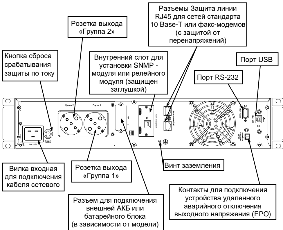
Рисунок 4 – Общий вид задней панели SKAT-UPS 2000-RACK-ON-4x9 P3, SKAT-UPS 2000-RACK-ON P3
