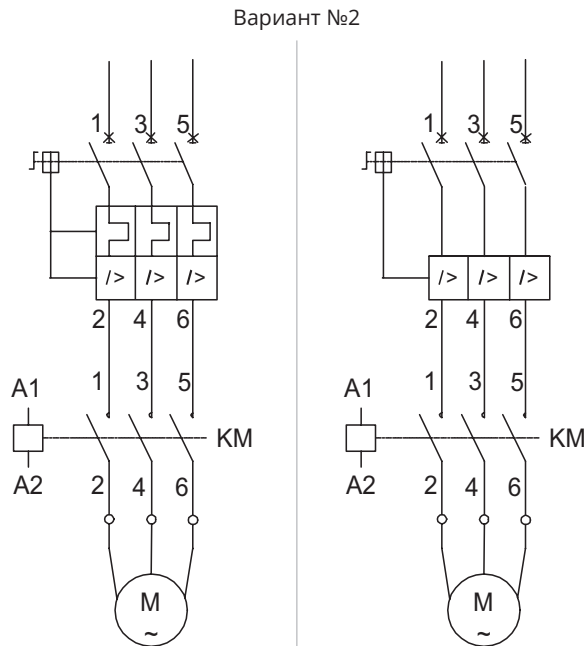
Подключение двигателя к ВА-450 через контактор
