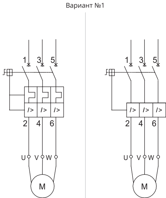
Подключение двигателя к ВА-450 напрямую
