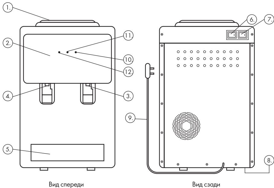
Вид спереди
