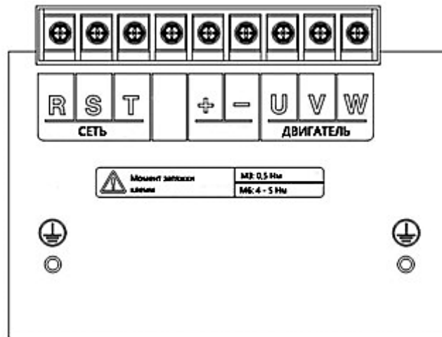
30, 37 кВт (040Н, 050Н)
