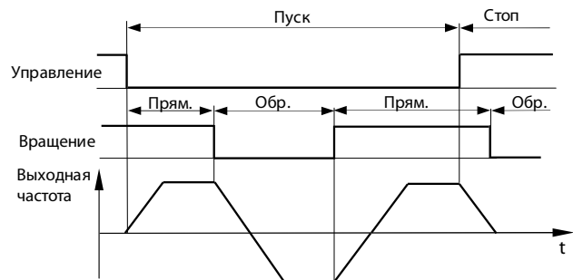
Рис.7.1б Двухпроводное управление F00.03=0, F04.19=0
