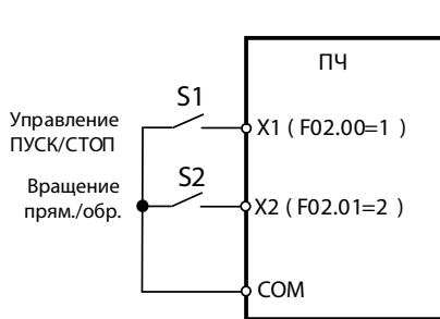
Рис.7.1а Двухпроводное управление F00.03=0
