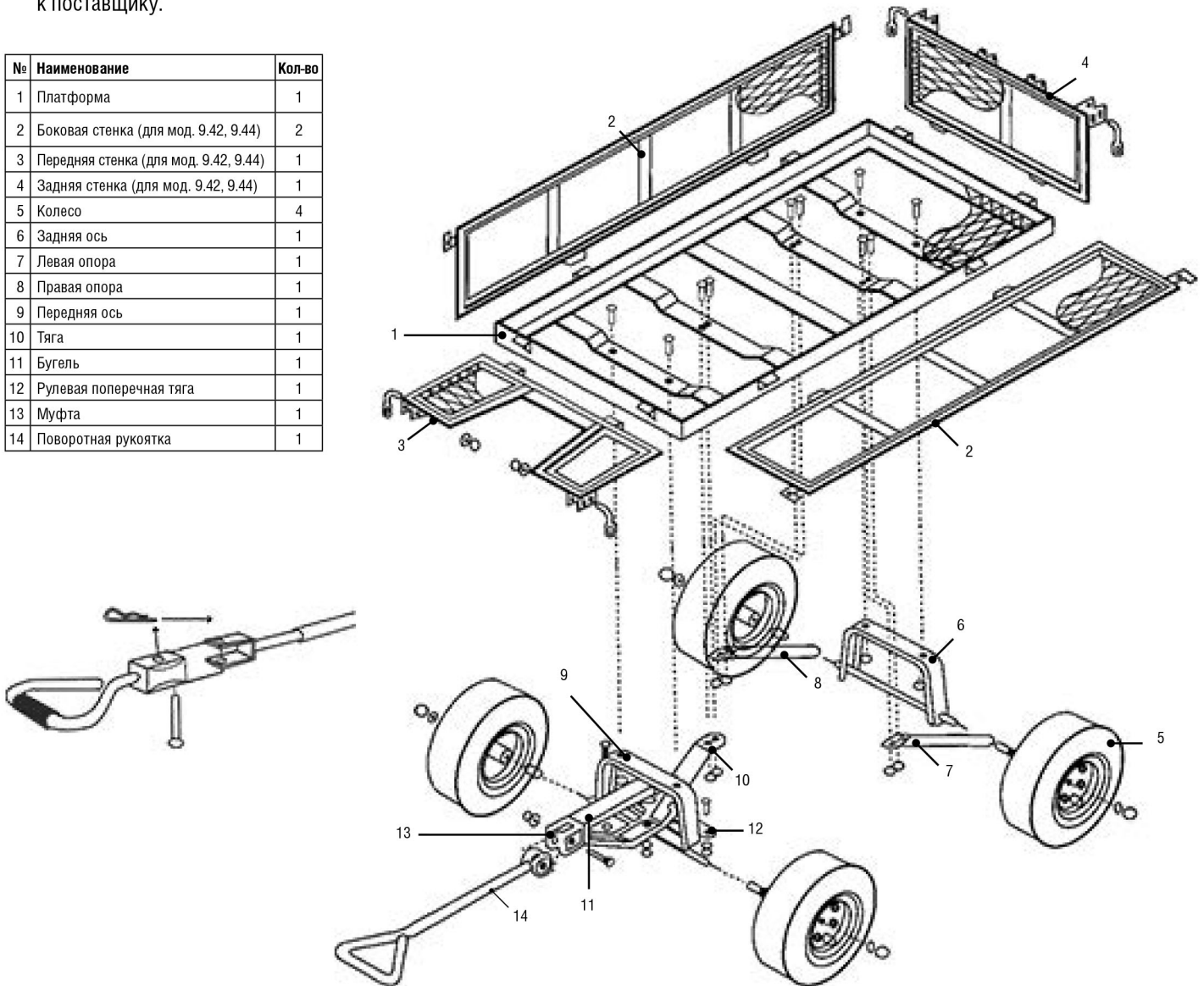
Рисунок 2 – Сборка тележки
